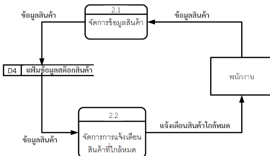
ภาพที่ 3.12 แผนภาพกระแสข้อมูล DFD 1 โปรเซสที่ 2 จัดการสต็อกสินค้า
