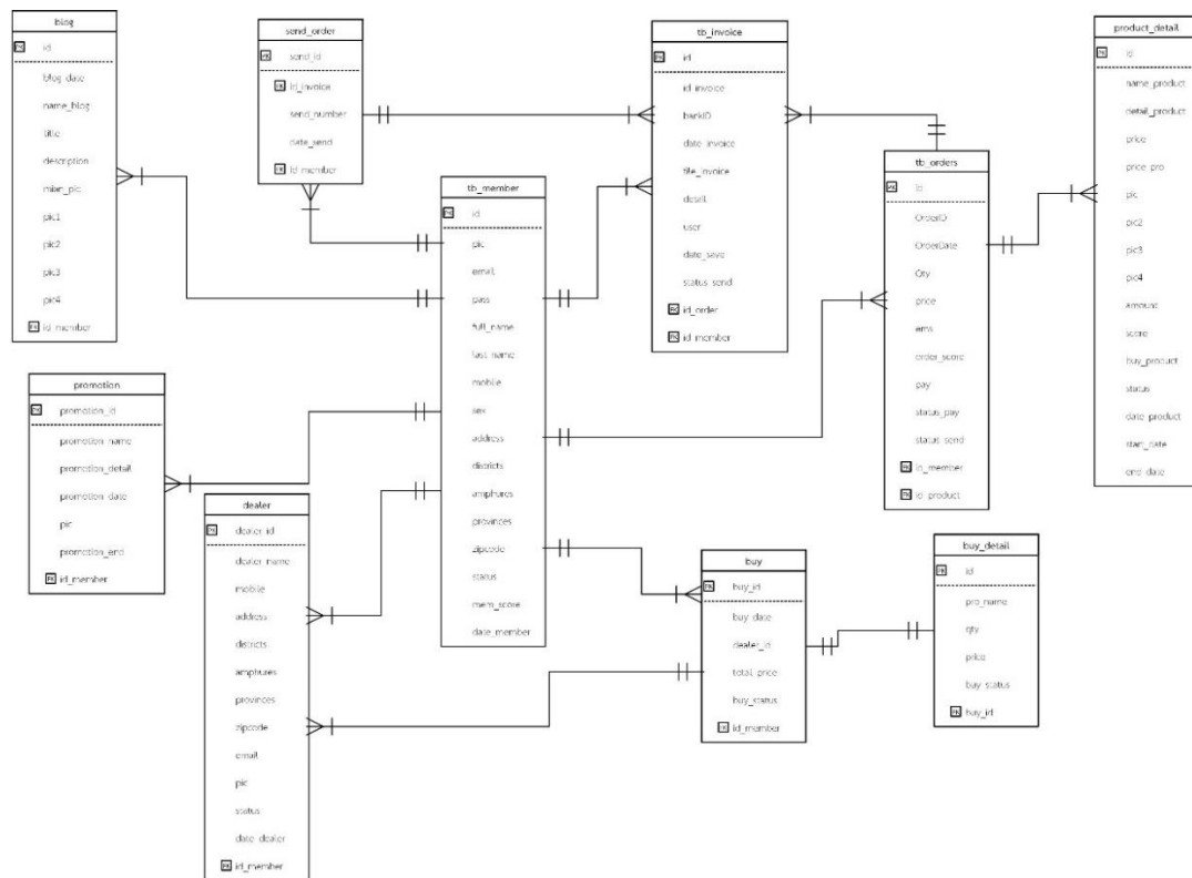
ภาพที่ 3.18 แสดงภาพความสัมพันธ์ของข้อมูลระบบบริหารจัดการห้างหุ้นส่วนจำกัด เจ. อาร์ แพทย์ภัณฑ์
