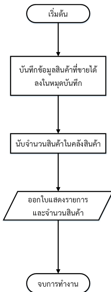
ภาพที่ 3.3 แสดงภาพ Flowchart ขั้นตอนการทำงานของคลังสินค้า
