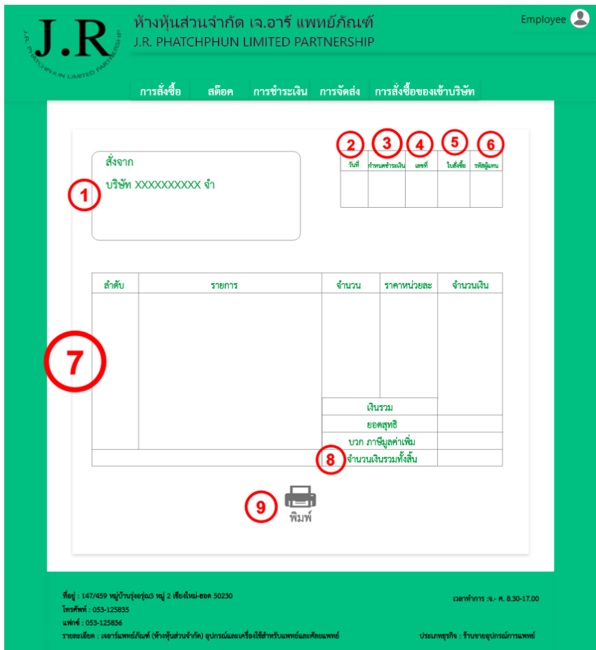
ภาพที่ 3.44 แสดงภาพหน้าจอใบสั่งซื้อของเข้าบริษัท
