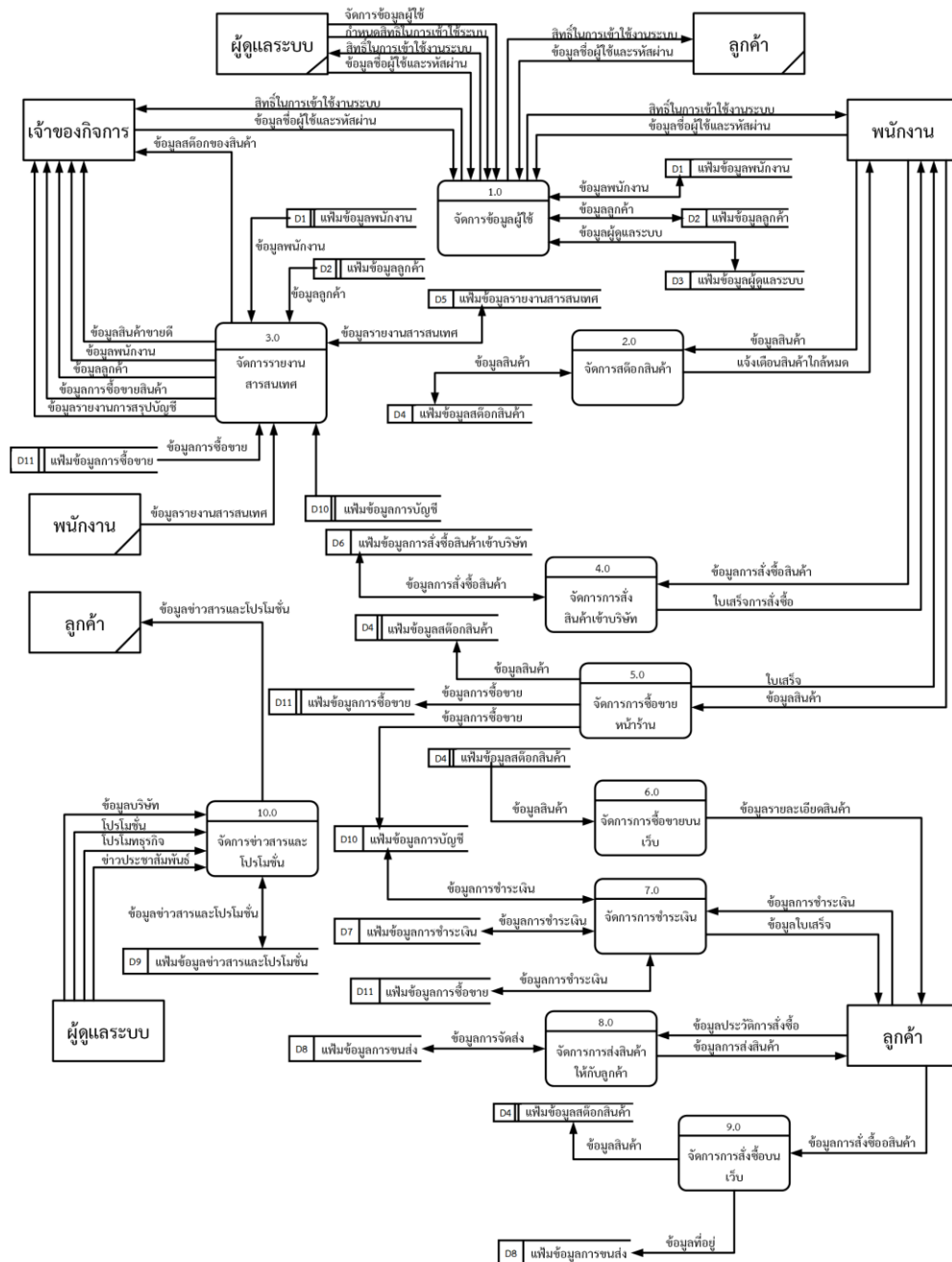
ภาพที่ 3.11 แผนภาพกระแสข้อมูลระดับที่ 0 ของระบบบริการจัดการรถจักรยานยนต์ เจ. อาร์ แพทย์ ภักดิ์
