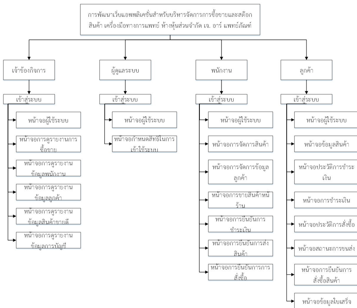
ภาพที่ 3.19 โครงสร้างระบบเว็บแอปพลิเคชันสำหรับบริหารจัดการการซื้อขายและสต็อก
