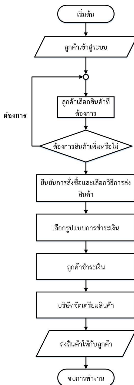
ภาพที่ 3.7 แสดงภาพ Flowchart ขั้นตอนการขายสินค้า
