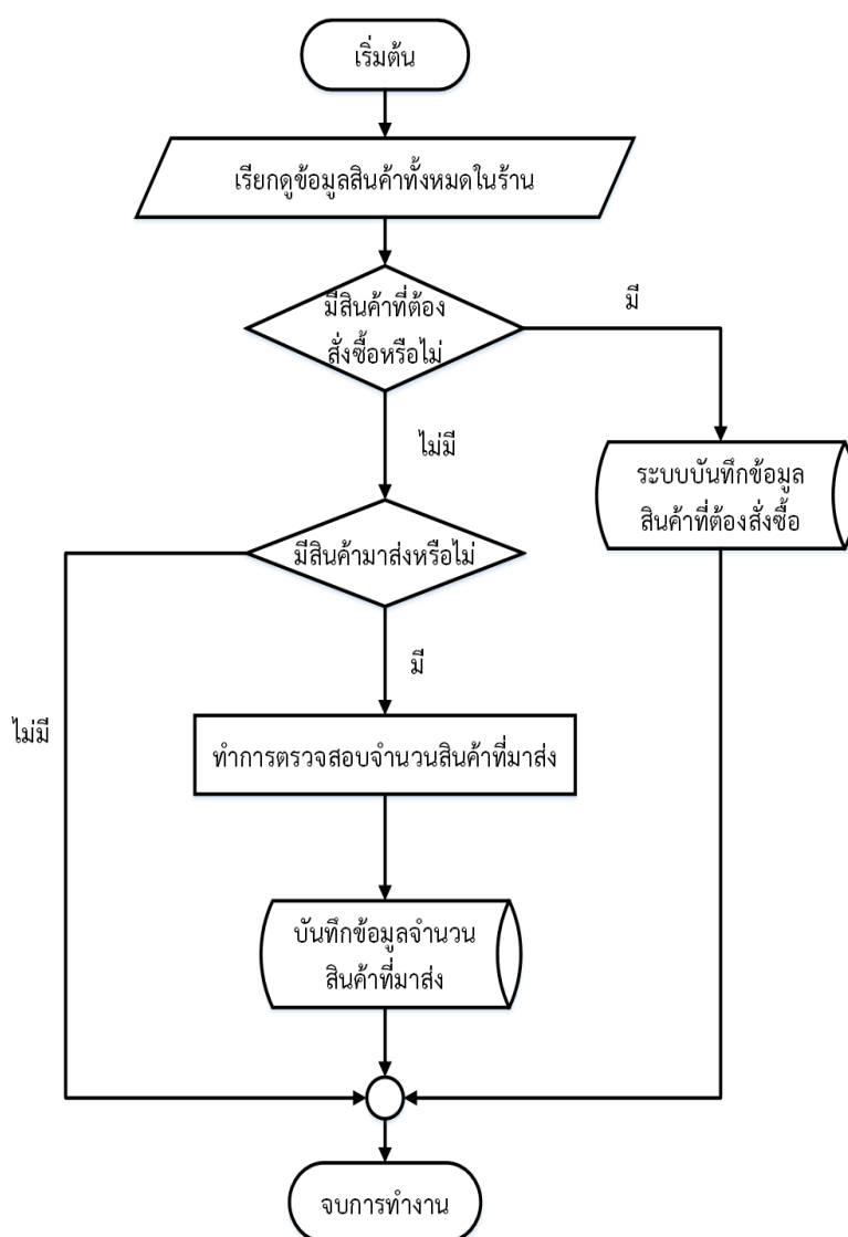
ภาพที่ 3.9 แสดงภาพ Flowchart ขั้นตอนการจัดการคลังสินค้า
