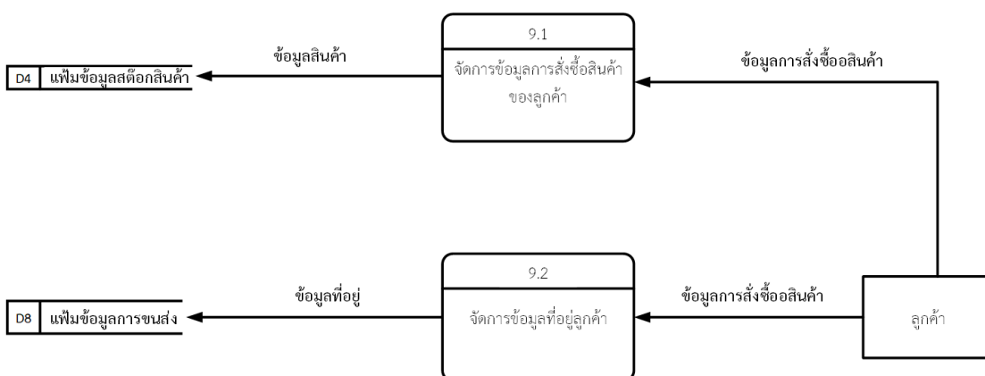
ภาพที่ 3.17 แผนภาพกระแสข้อมูล DFD 1 โปรเซสที่ 9 จัดการข้อมูลการสั่งซื้อสินค้าบนเว็บ
