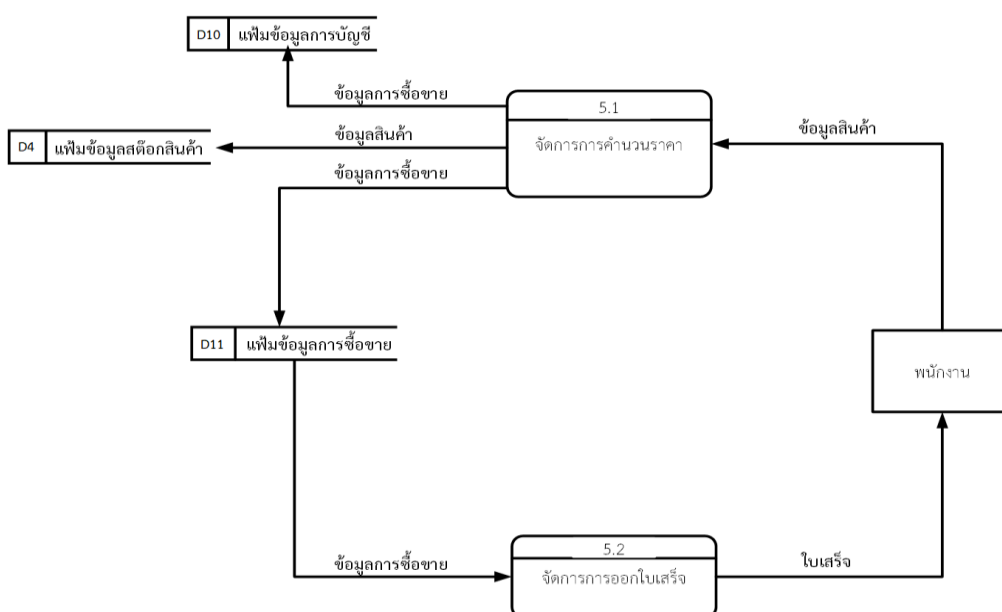
ภาพที่ 3.14 แผนภาพกระแสข้อมูล DFD 1 โปรเซสที่ 5 จัดการข้อมูลการซื้อขายหน้าร้าน
