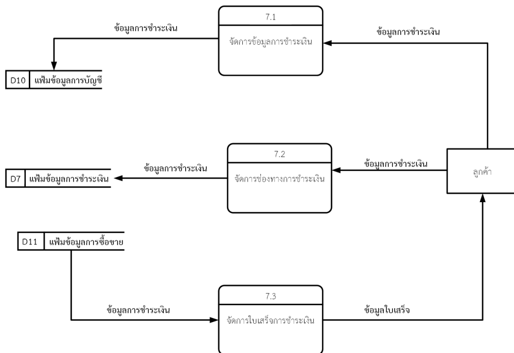
ภาพที่ 3.15 แผนภาพกระแสข้อมูล DFD 1 โปรเซสที่ 7 จัดการข้อมูลการชำระเงิน
