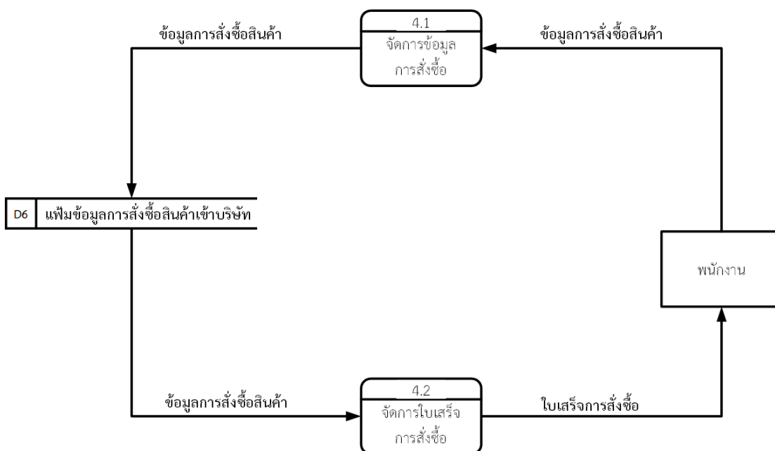
ภาพที่ 3.13 แผนภาพกระแสข้อมูล DFD 1 โปรเซสที่ 4 จัดการข้อมูลการสั่งซื้อสินค้าเข้าบริษัท
