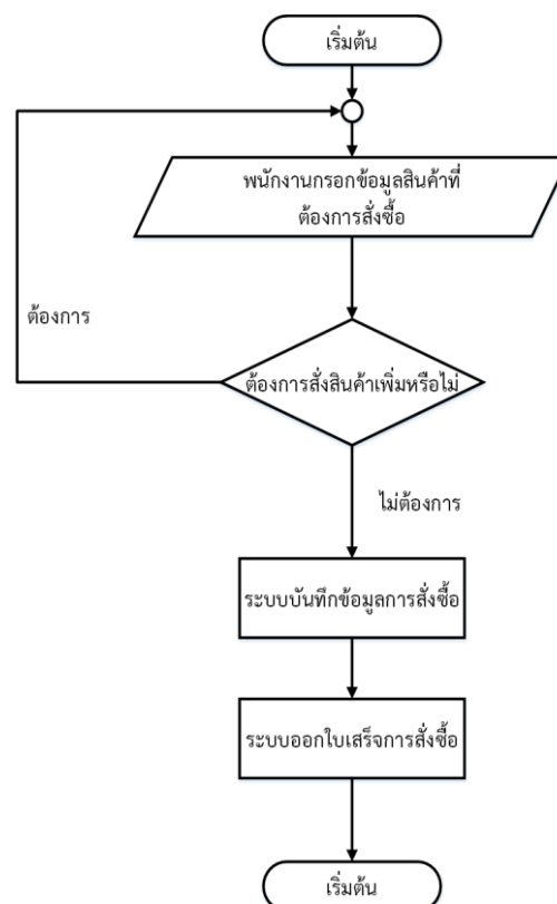
ภาพที่ 3.8 แสดงภาพ Flowchart ขั้นตอนการจัดการสั่งซื้อสินค้า
